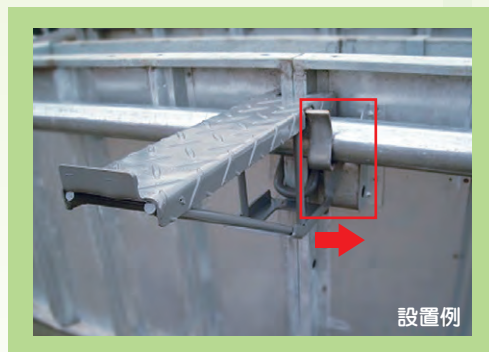
※50単管パイプ受は右側に寄せて取り付けして下さい。
