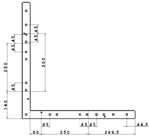
8121376 定規 コーナーM用 0.5P 120巾 (601mm)
