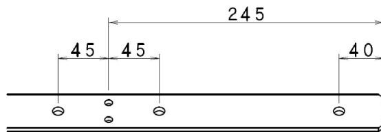
8121369 定規 直線M用 1.0P (990mm)
