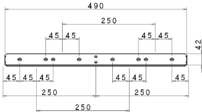
8121371 定規 直線M用 0.5P (490mm)
