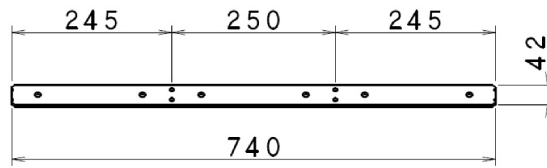
8121370 定規 直線M用 0.75P (740mm)
