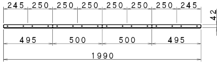
8121368 定規 直線M用 2.0P (1990mm)
