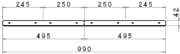
8121369 定規 直線M用 1.0P (990mm)
