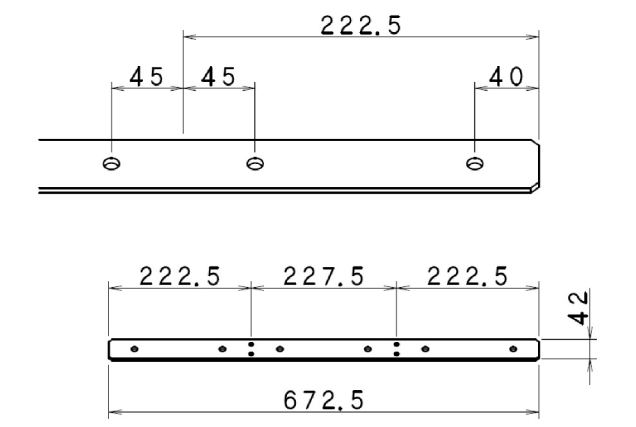
8121374 定規 直線尺用 0.75P (672.5mm)
