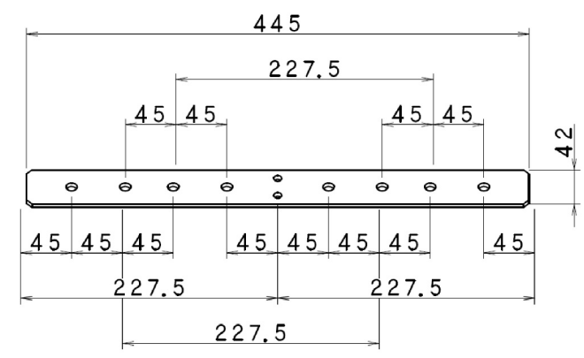
8121375 定規 直線尺用 0.5P (445mm)
