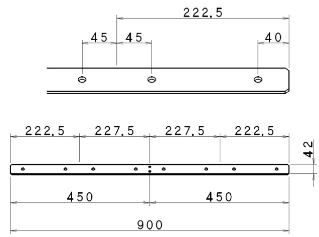
8121373 定規 直線尺用 1.0P (900mm)
