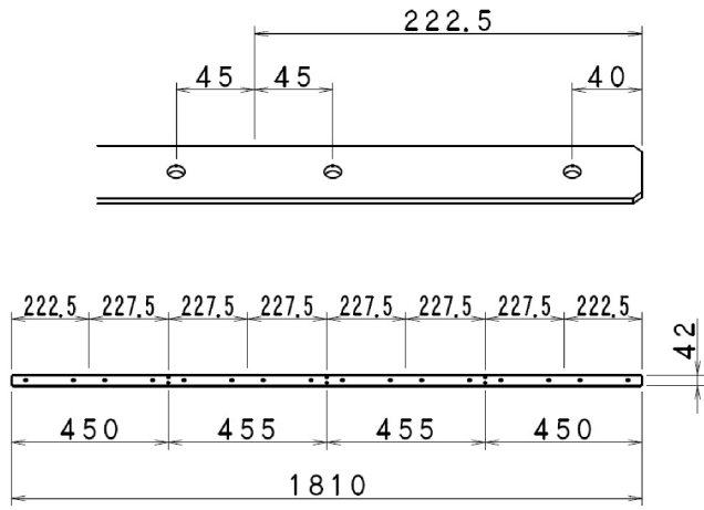
8121372 定規 直線尺用 2.0P (1810mm)
